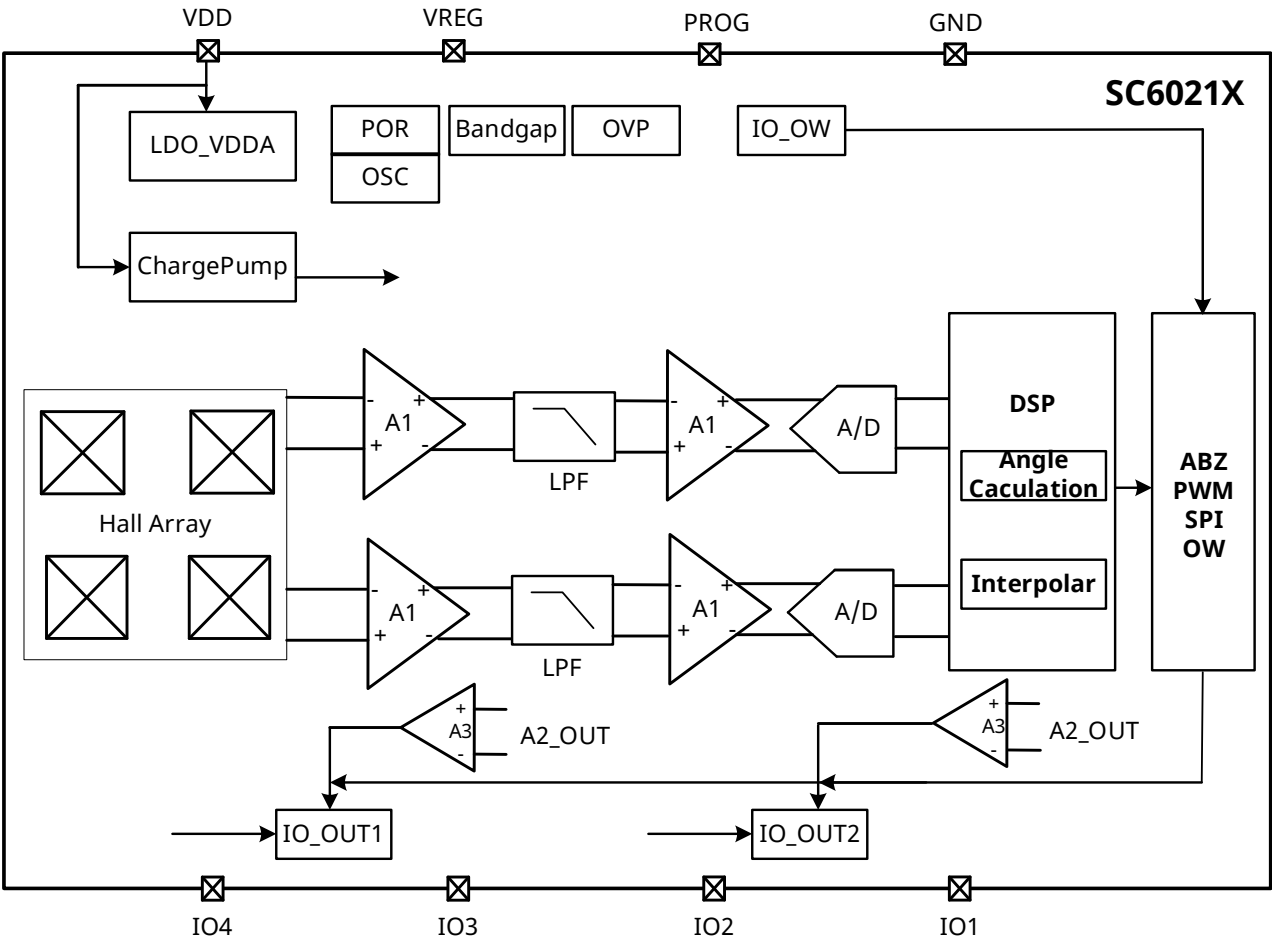
图 3 功能框图
